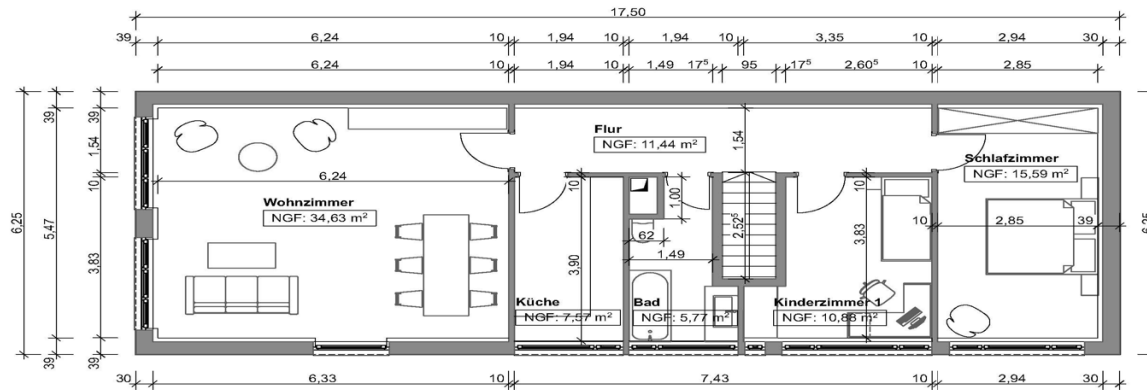
Grundriss 1.OG M.1:100
