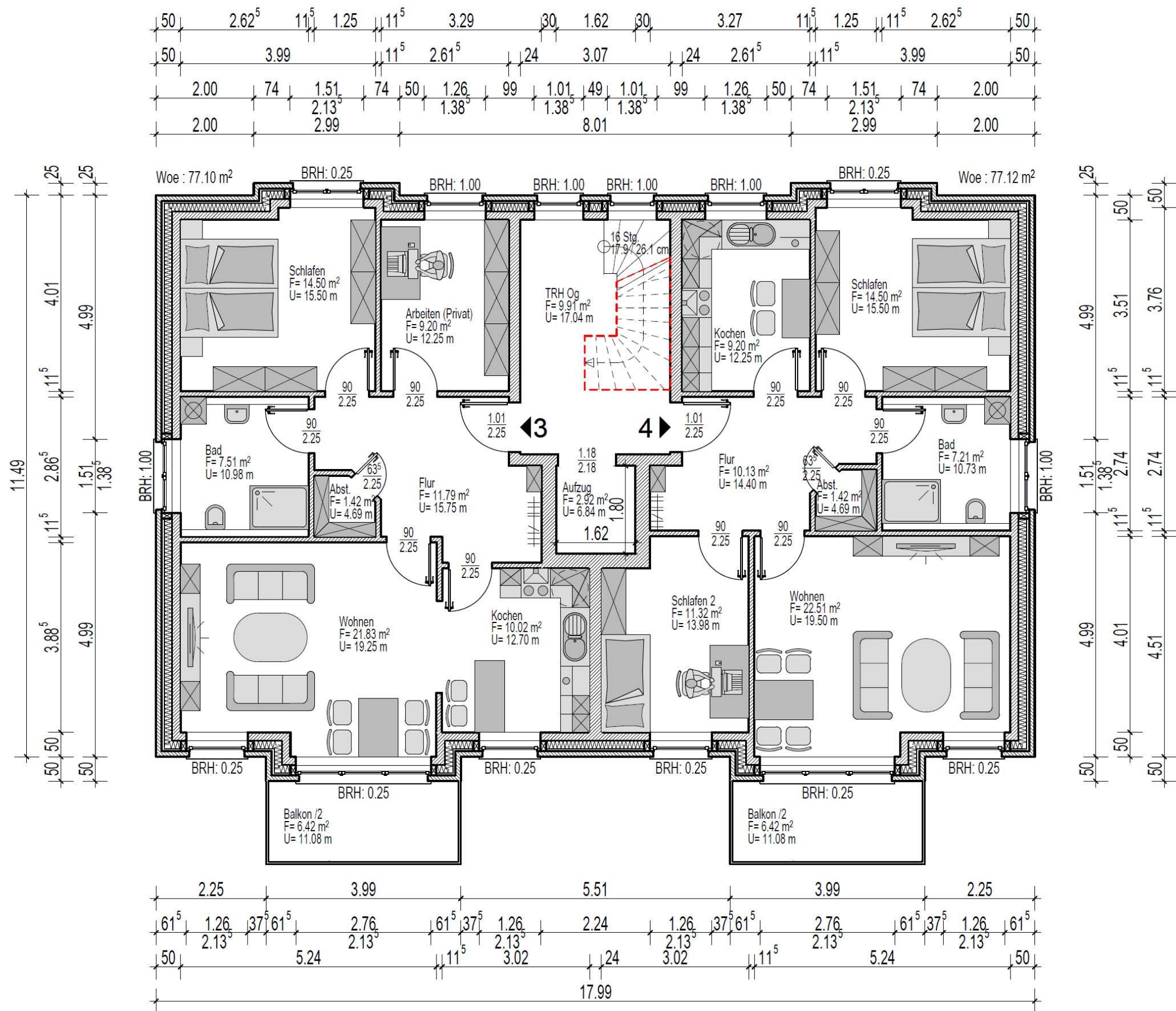
Obergeschoss - Grundriss
