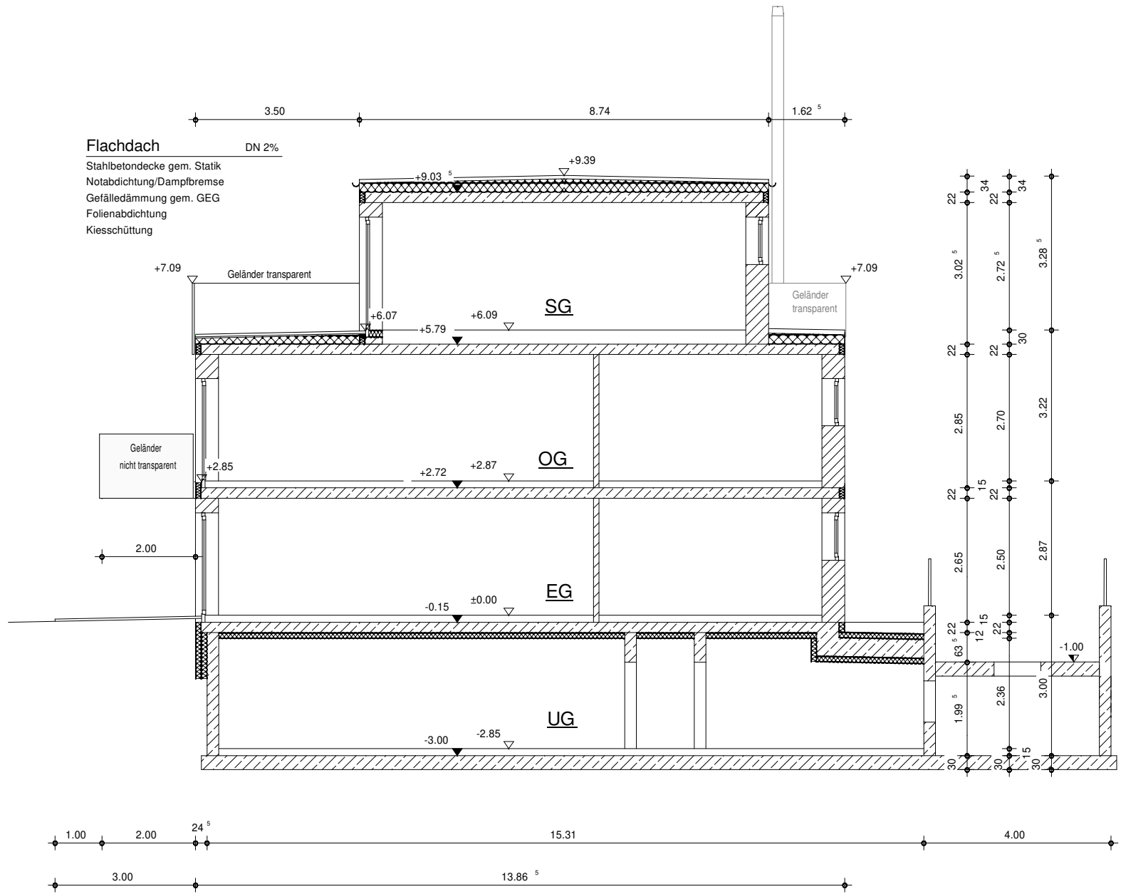
SCHNITT Haus Ost
