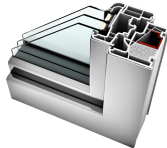
KUNSTSTOFF-ALU FENSTER
