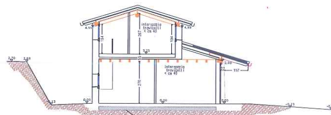
SEZIONE A-A
