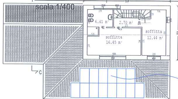
PIANO PRIMO
