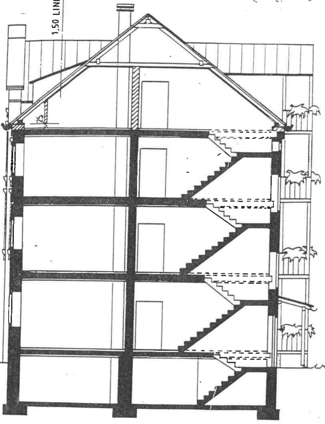
SCHNITT A-A
