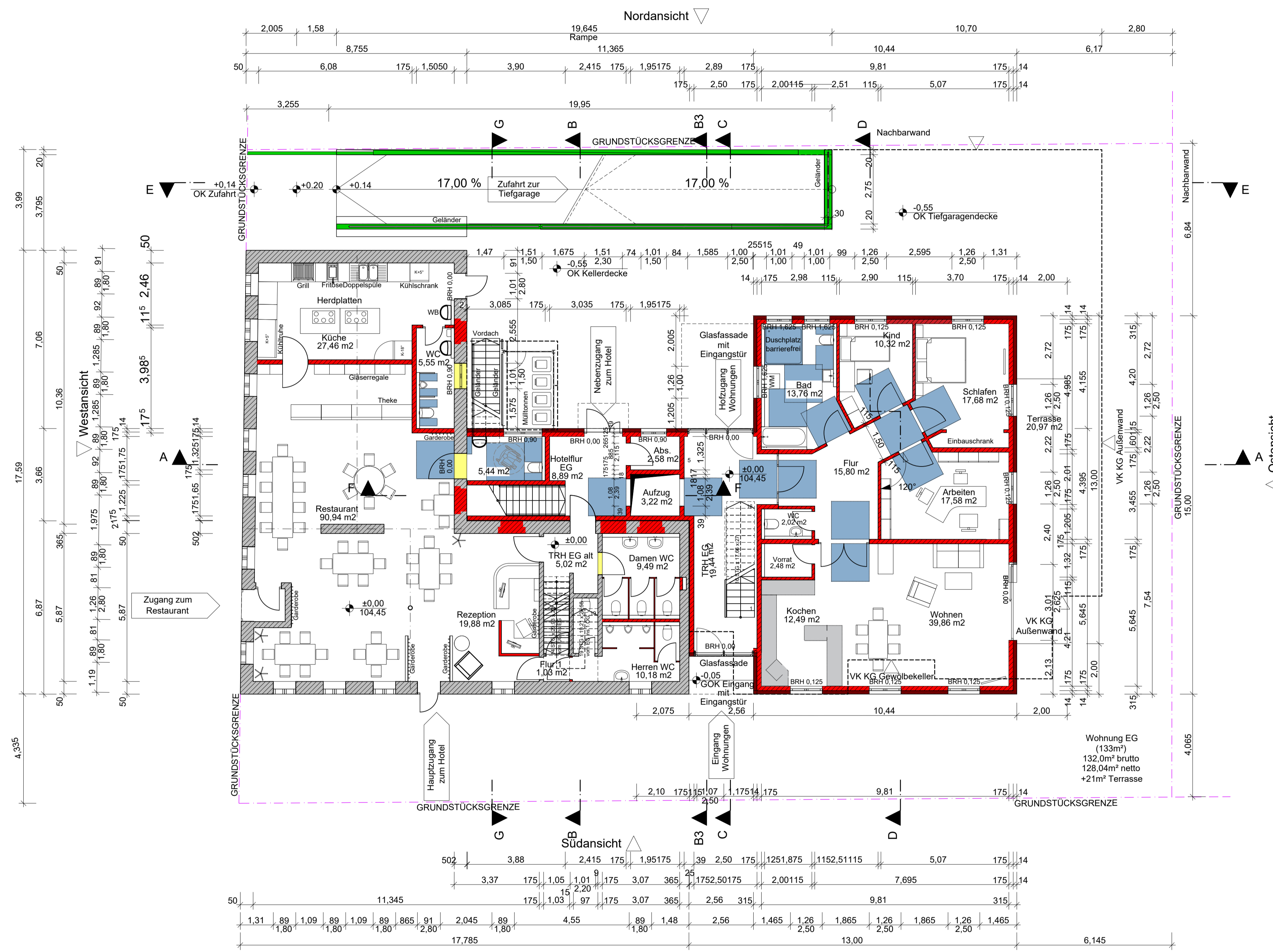
EG Alt- und Neubau 0,00m
