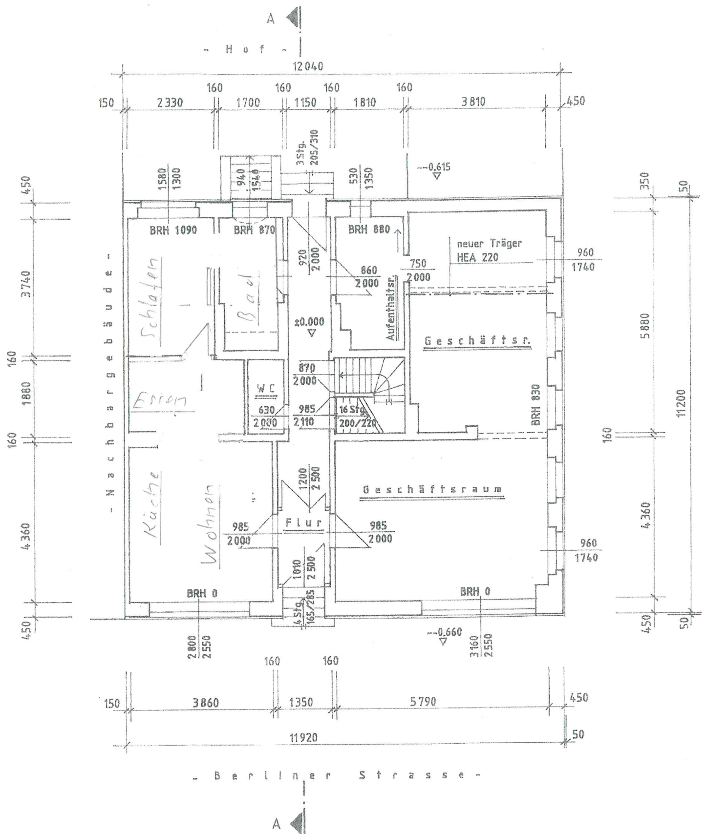
Berliner Straße 25 16303 Schwedt Grundriss - Erdgeschoss
