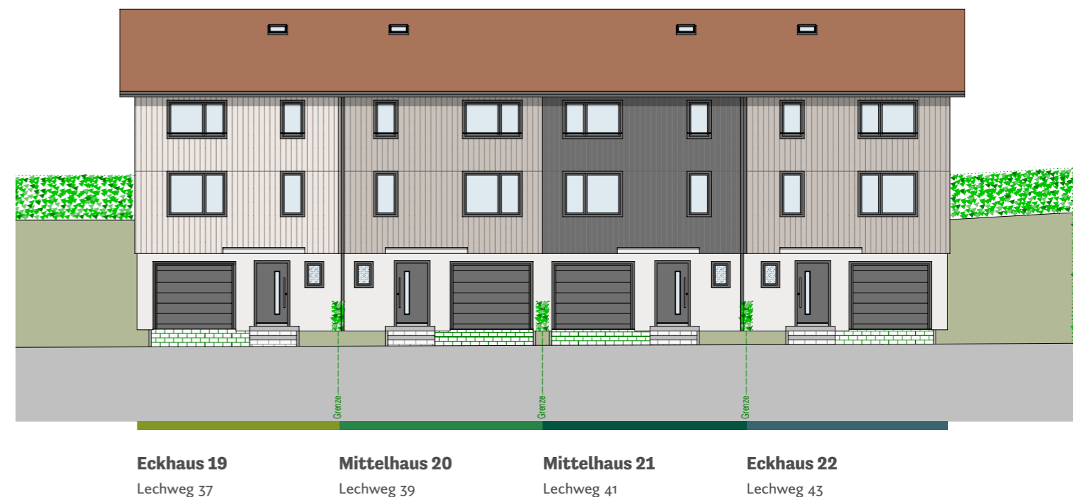
Nord-Ost-Ansicht
