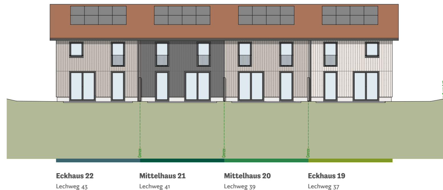
Süd-West-Ansicht
