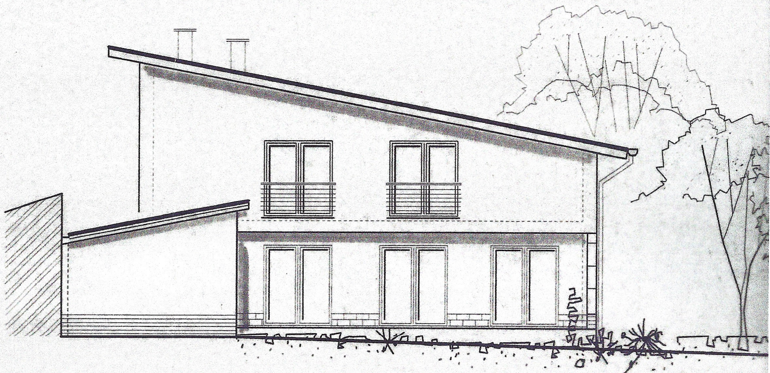
Ansicht Osten
