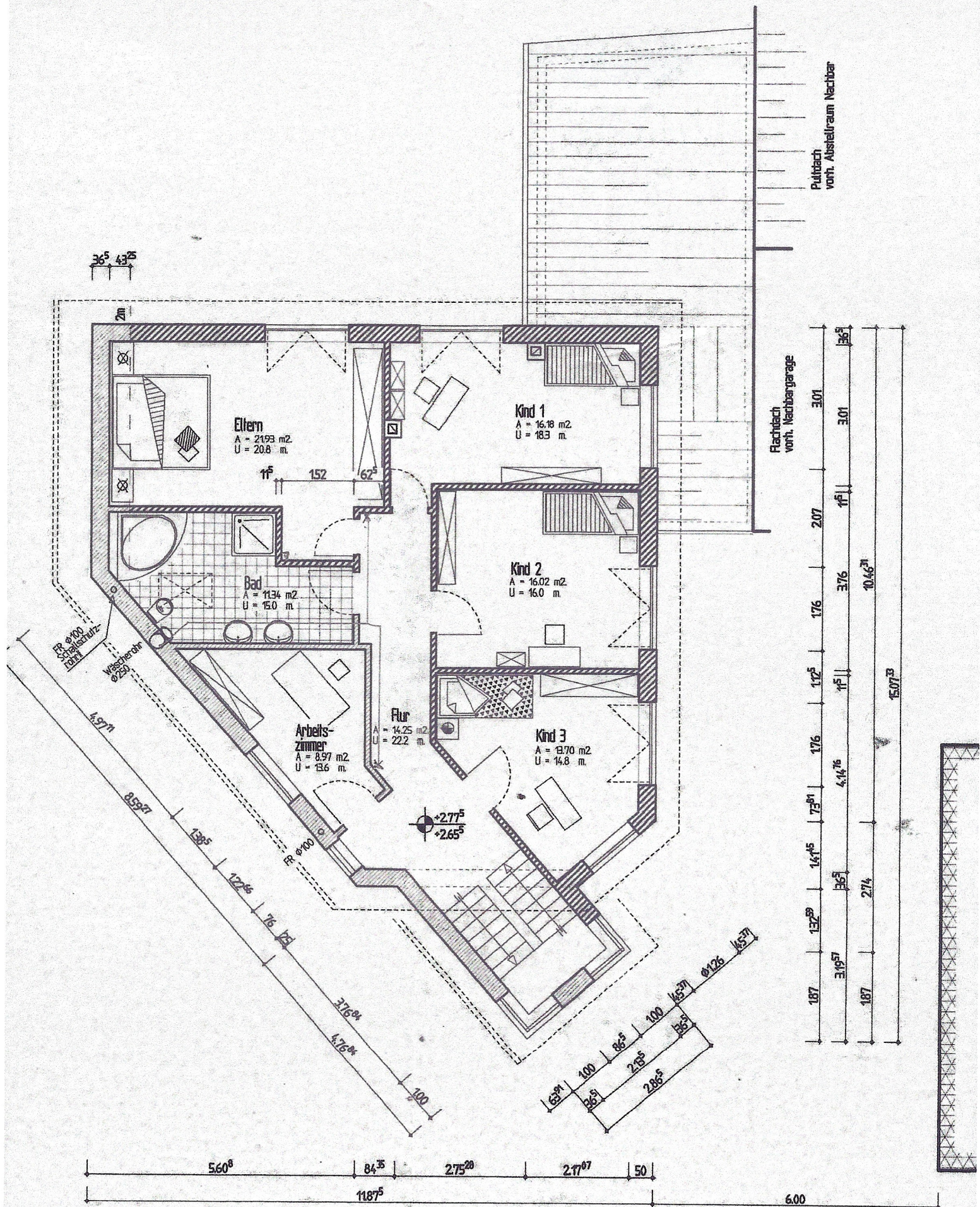
Grundriss Dachgeschoss
