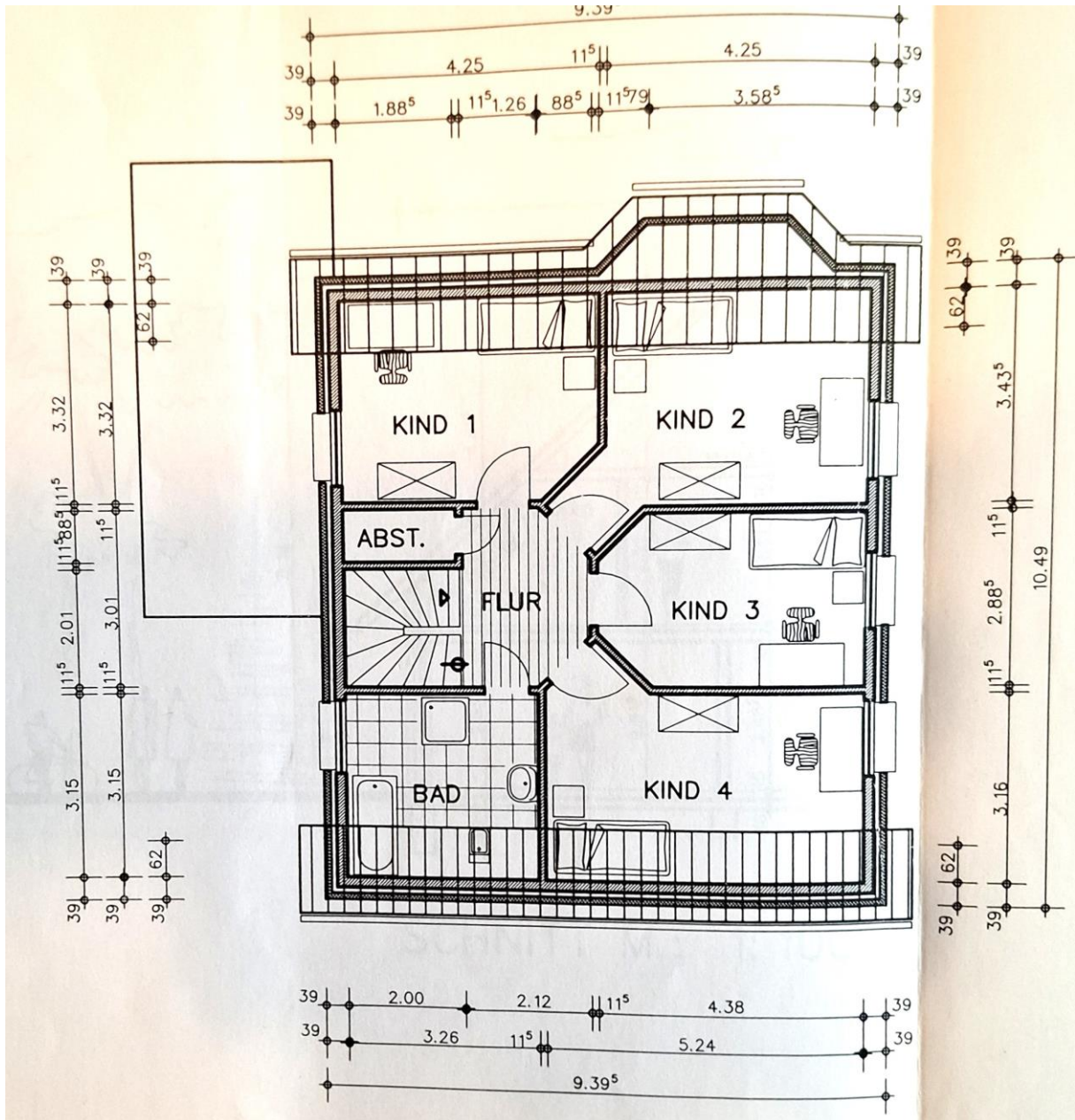
DACHGESCHOSS M.: 1:100
