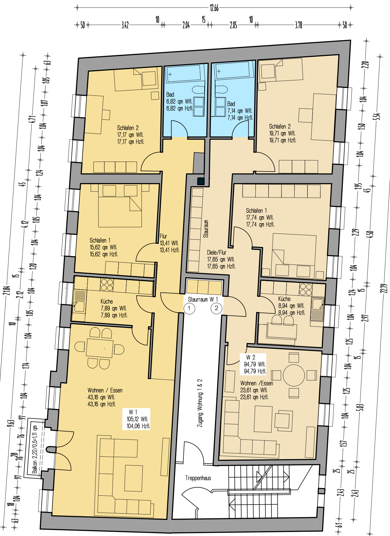
Wohnung 1 & 2 - 1 OG - Kirchstr. 20
