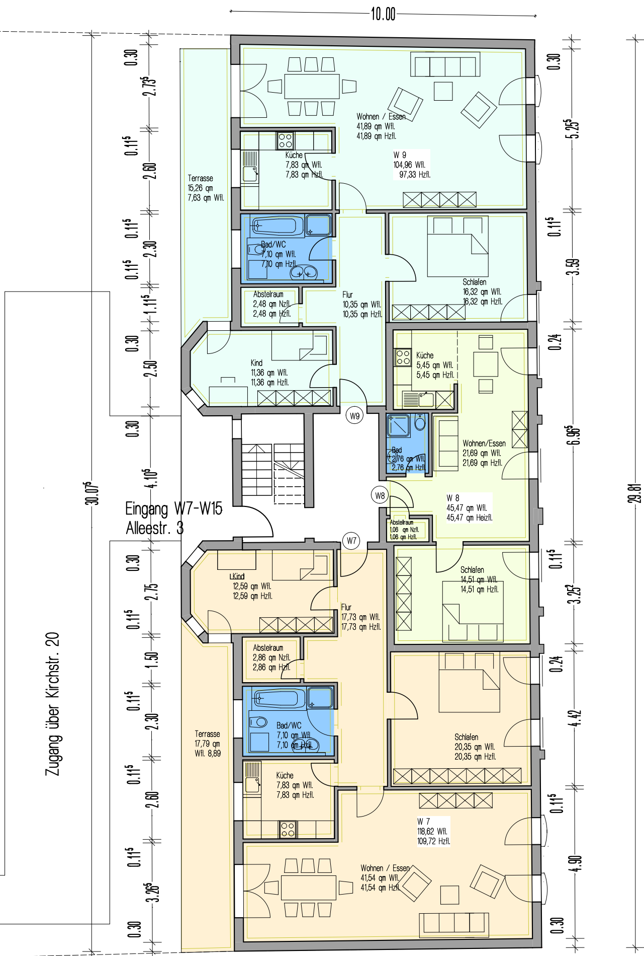
Wohnung 7 - 8 - 9 1 OG Alleestr. 3 M 1 : 125
