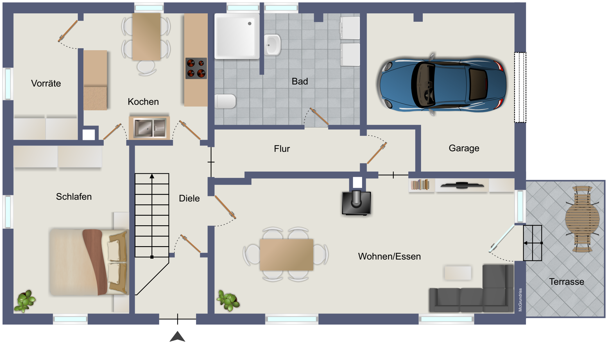
Erdgeschoss
