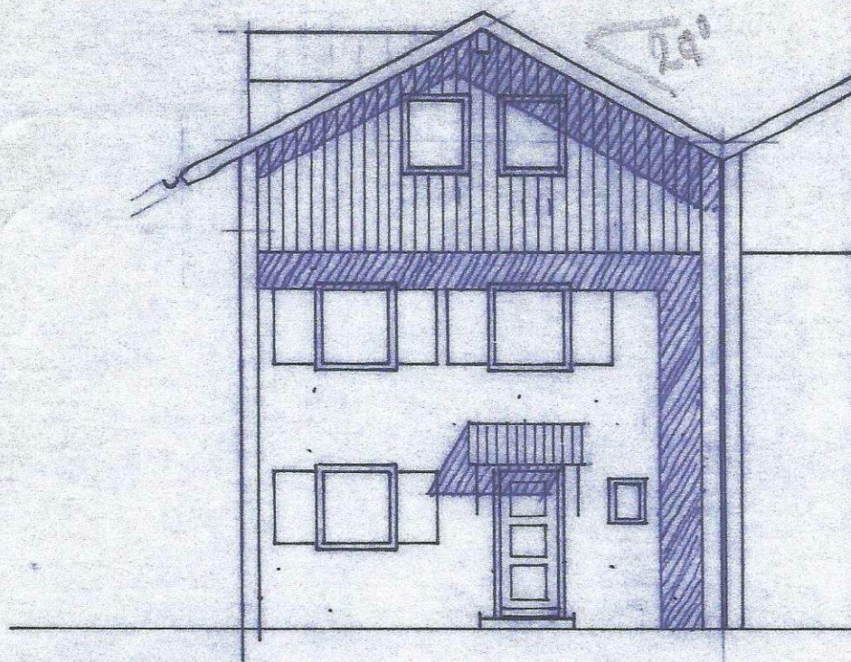
NORDANSICHT
