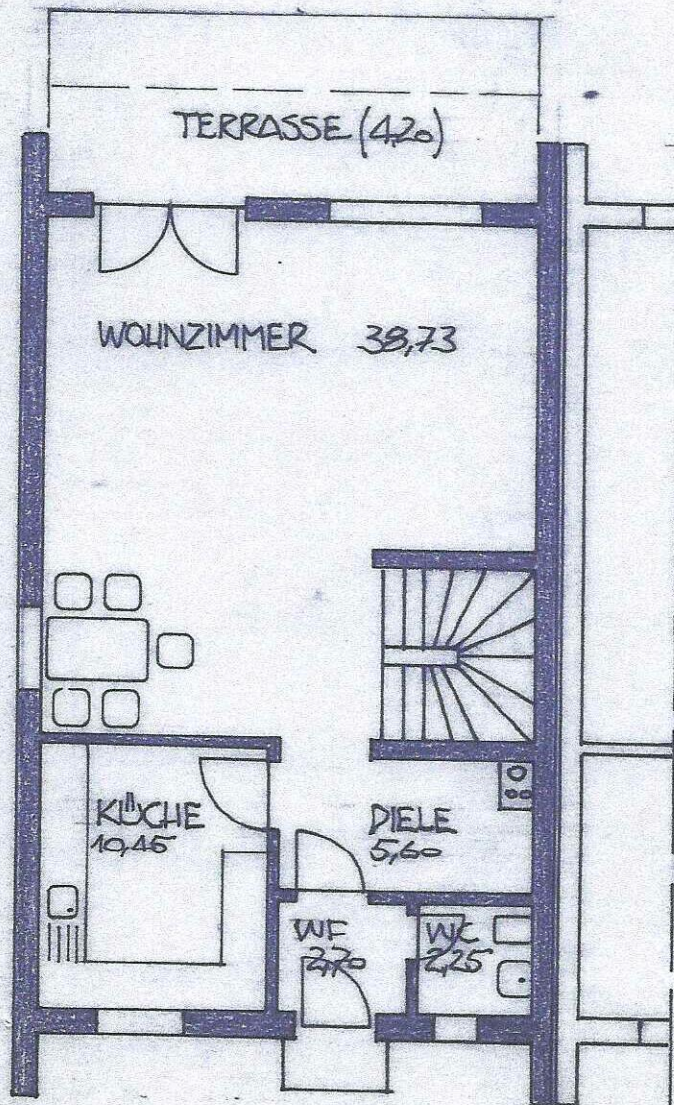
ERDGESCHOSS
