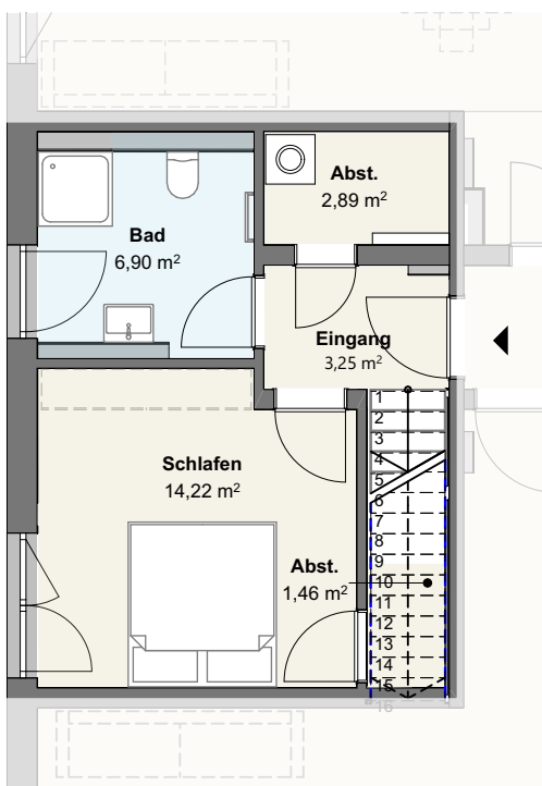
Obergeschoss
