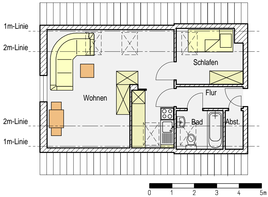
Typengrundriss
