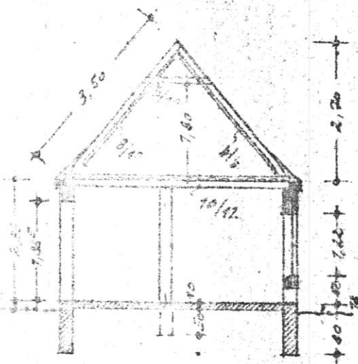
SEHNITT
