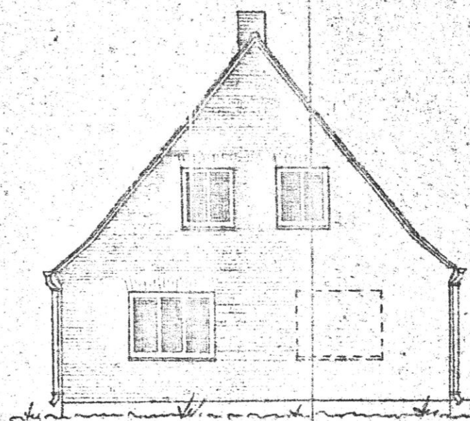
GIEBELANSICHT 2. Bauabschnitt
