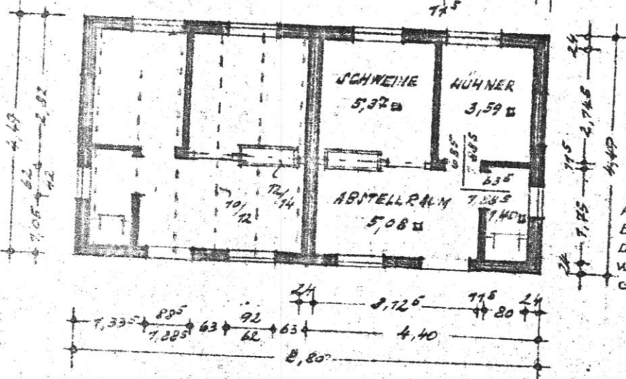
GRUNDRISS
