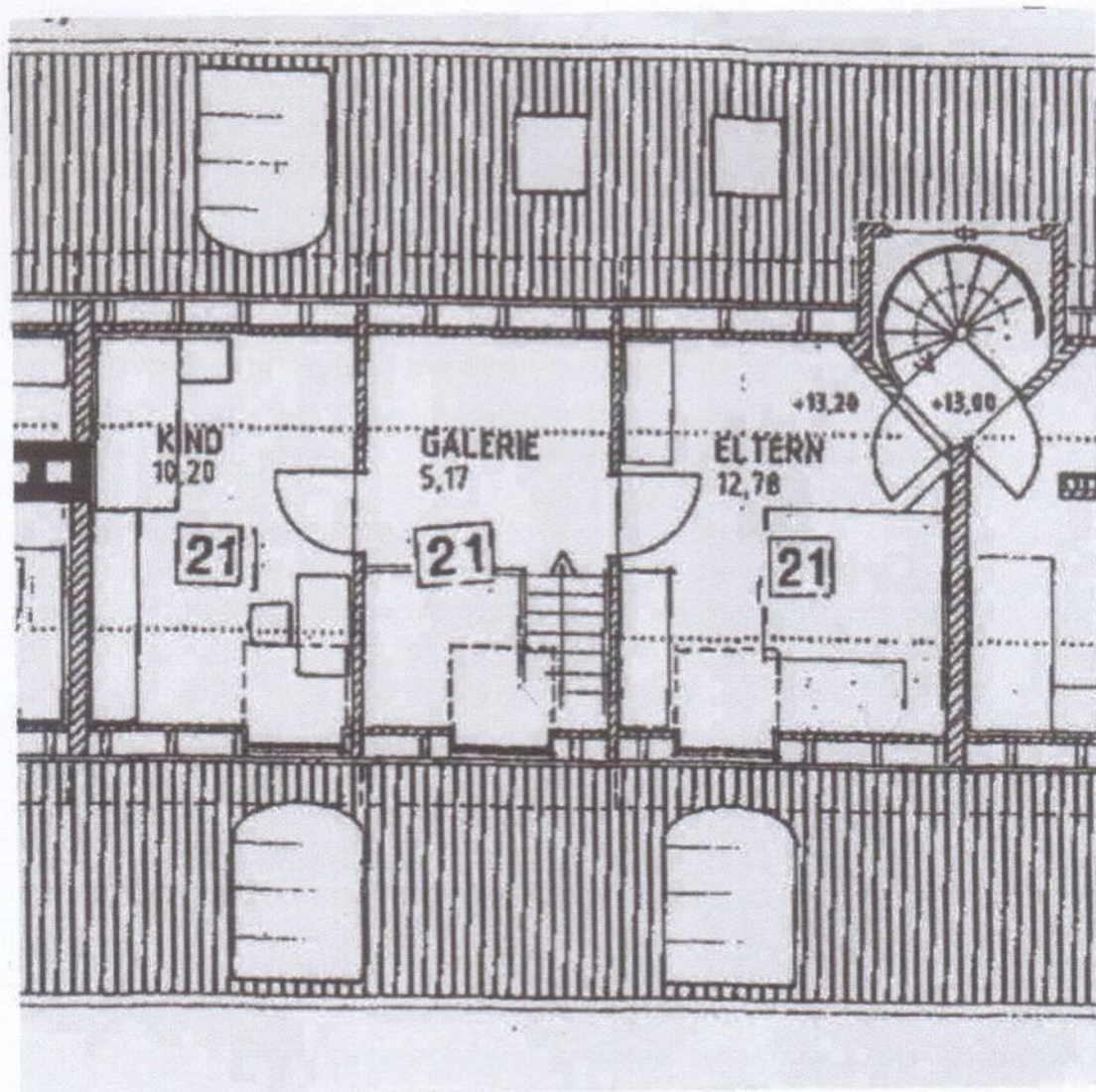
2. Dachgeschoss
