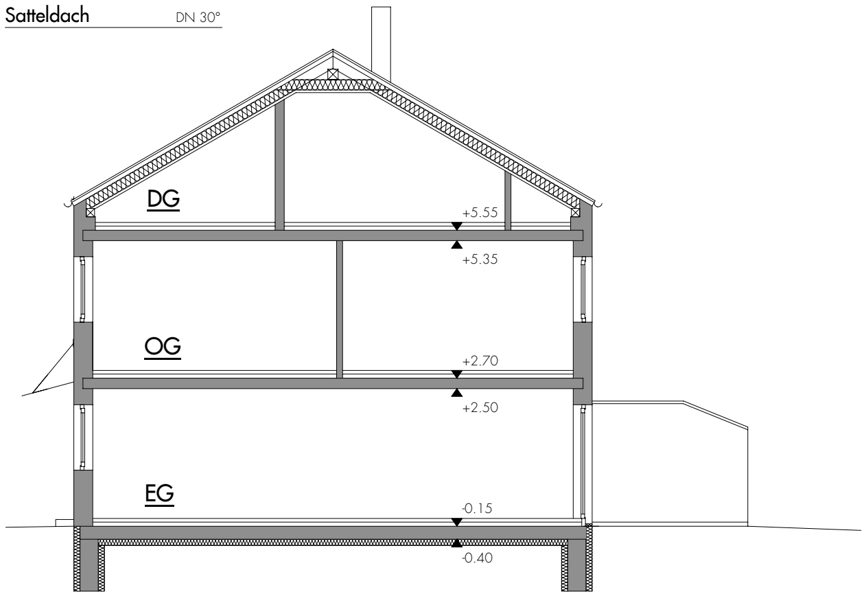
SCHNITT A-A EXPOSÉ
