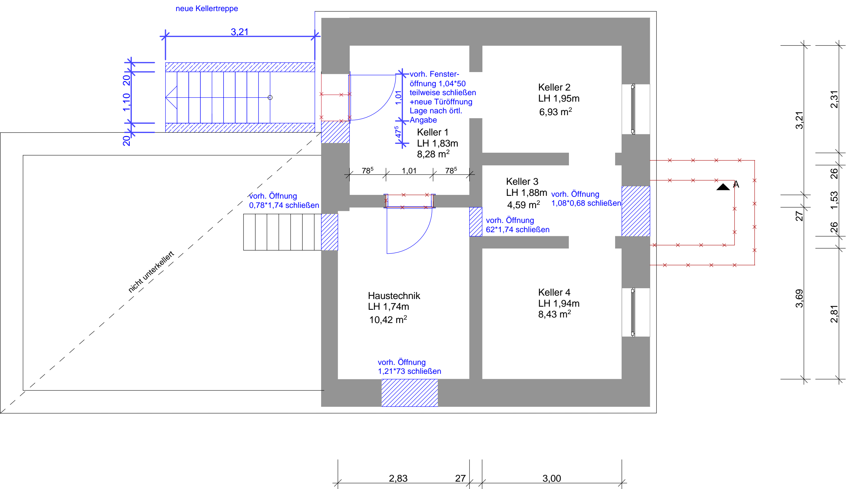
Grundriss Kellergeschoss
