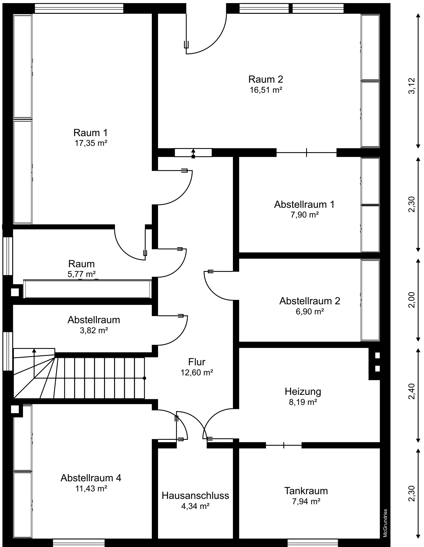
Keller/Gartengeschoss
