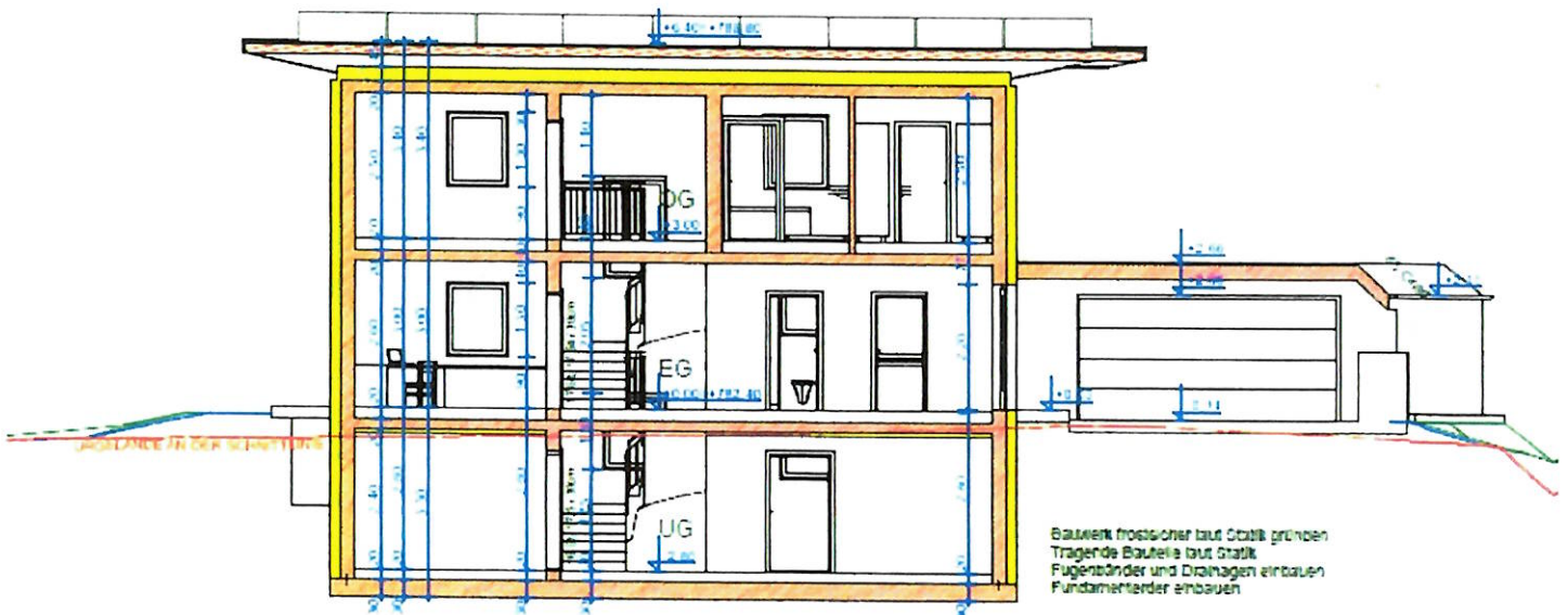
SCHNITT A - A
