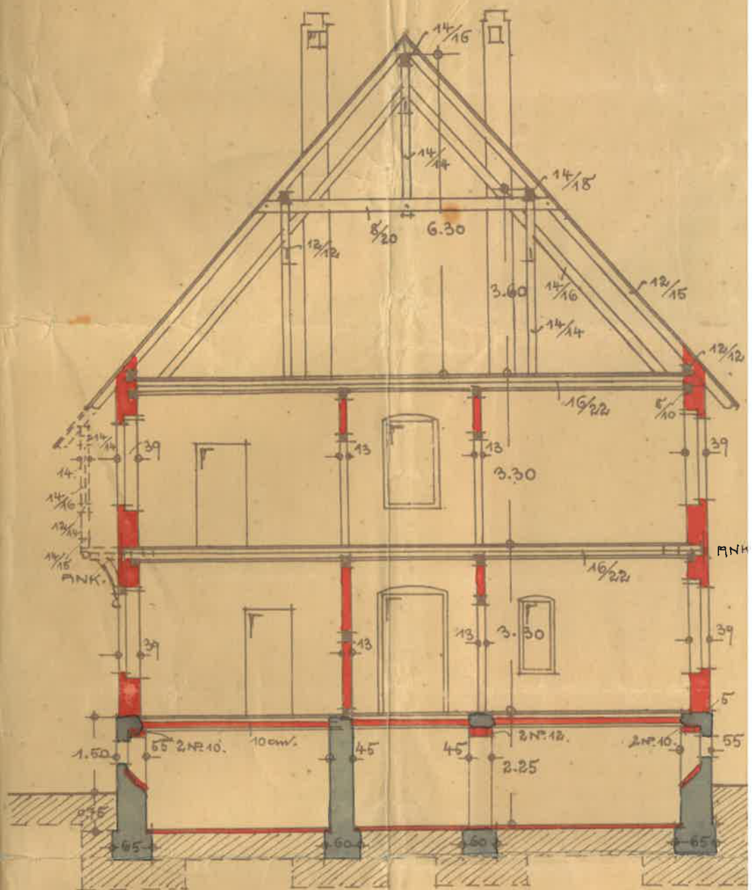
— SCHNITT A-B. —
