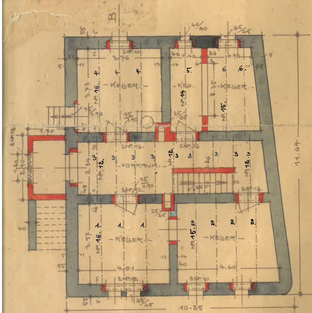
— KELLERGE5CHO55. —
