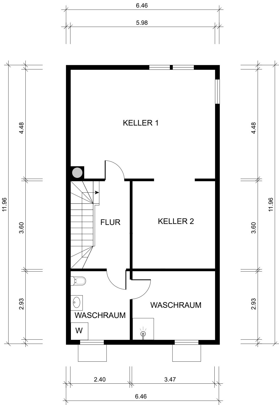
UNTERGESCHOSS
