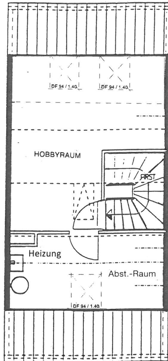
Dachgeschoss
