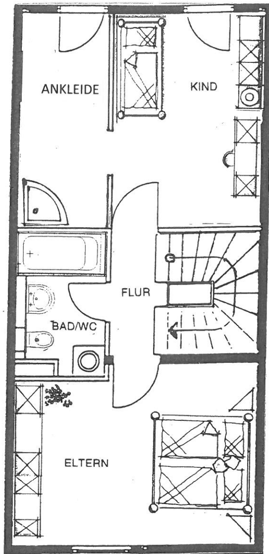
Obergeschoss
