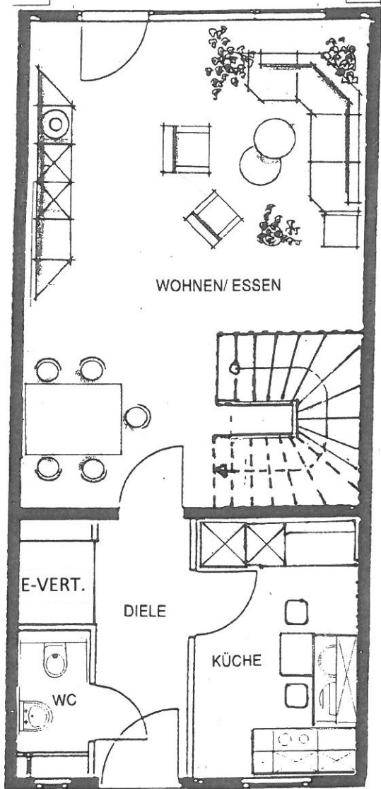
Erdgeschoss
