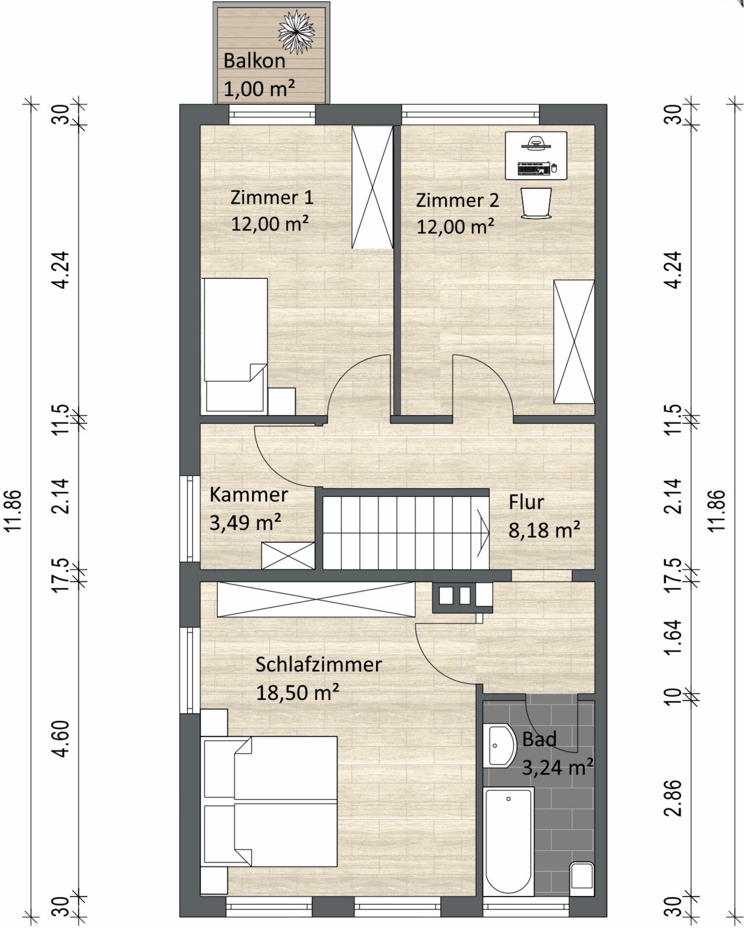
3-Zimmer-Variante
