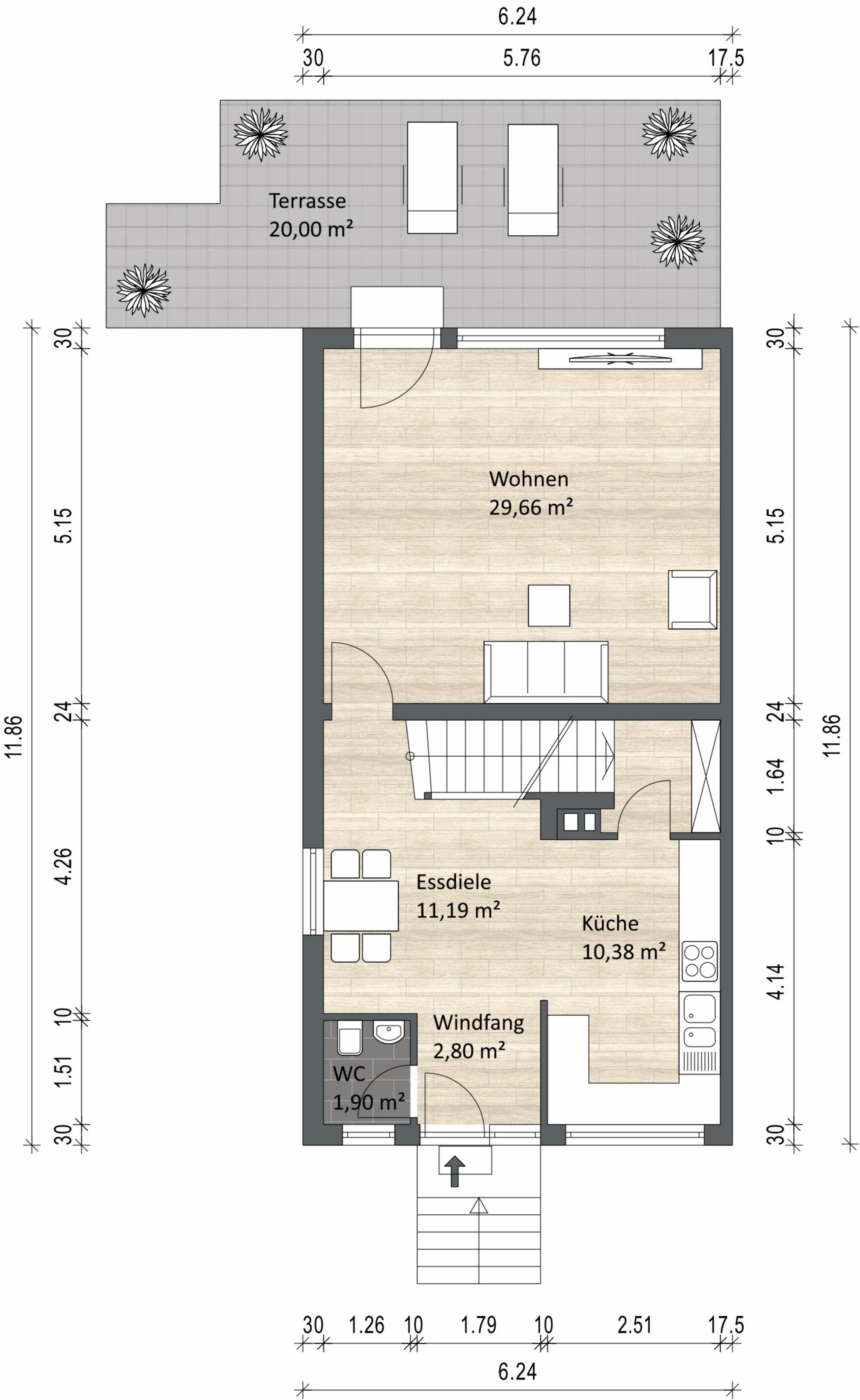
Erdgeschoss
