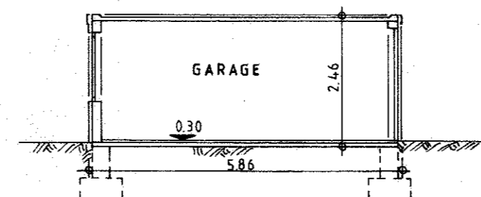
SCHNITT C-C
