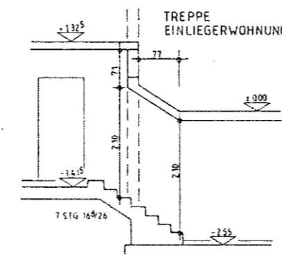
SCHNITT B-B
