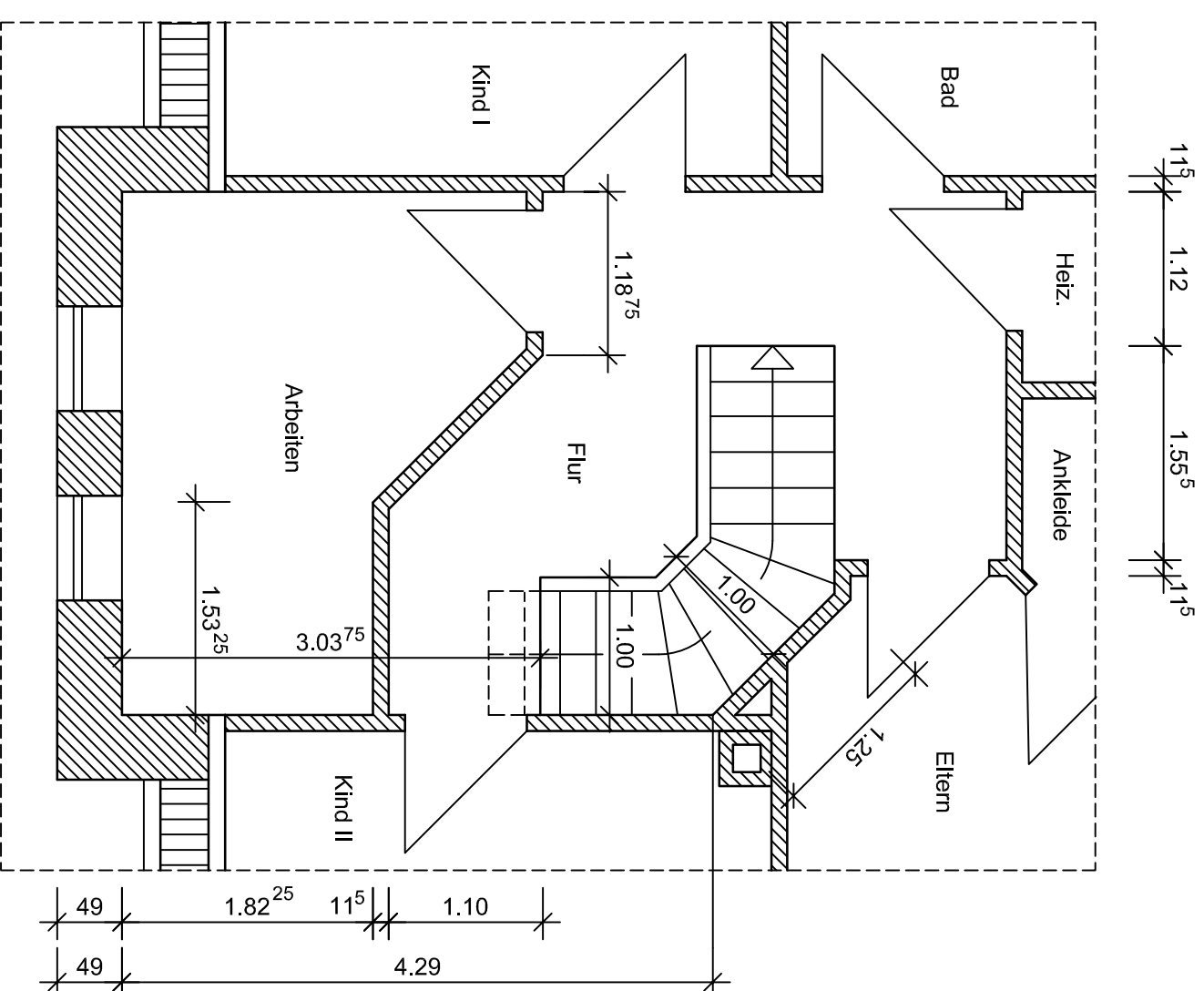
Ausschnitt Flur M. 1:50
