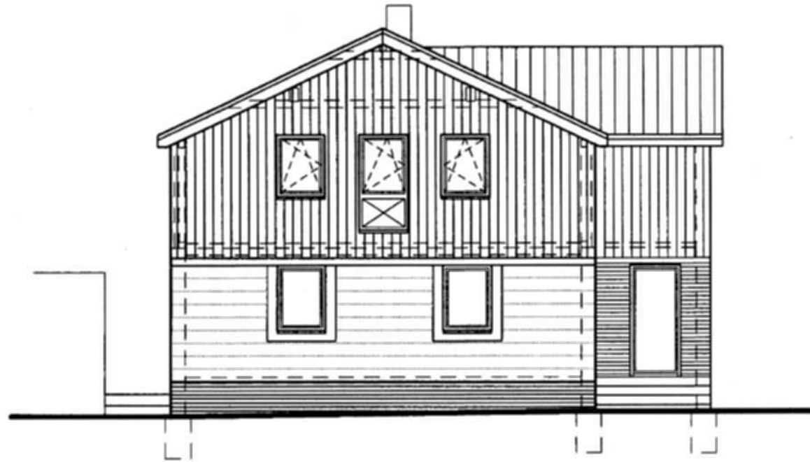
NORD-WEST-ANSICHT VARIANTE A
