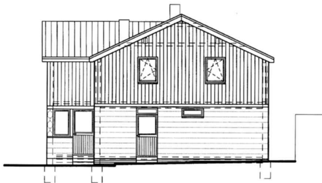
SUD-OST-ANSICHT
