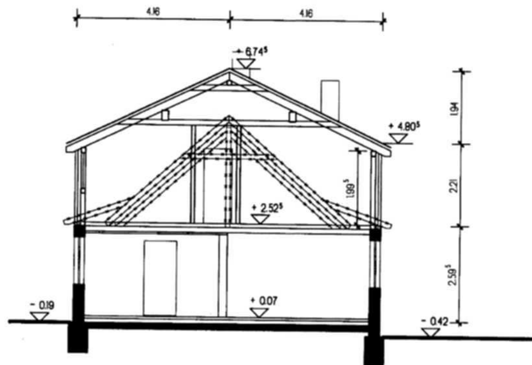
SCHNITT A-A
