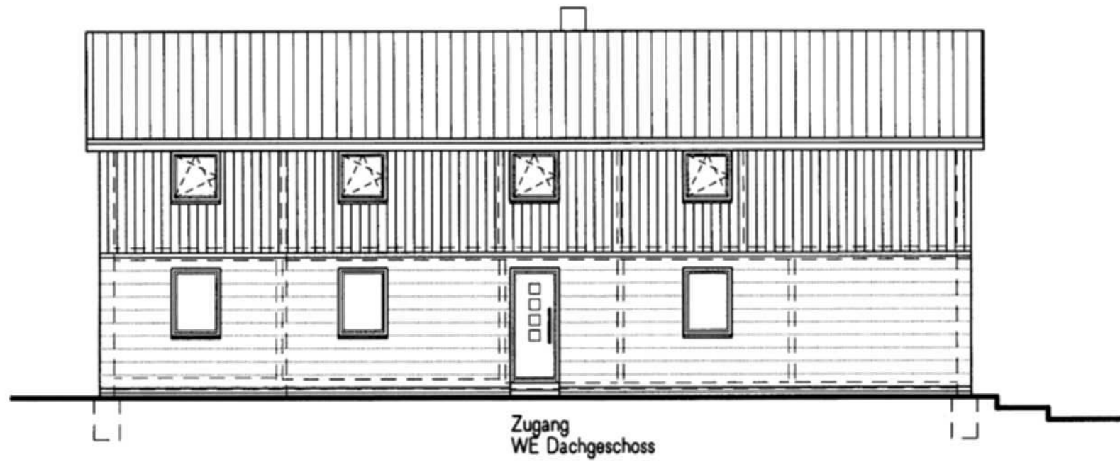
NORD-OST-ANSICHT
