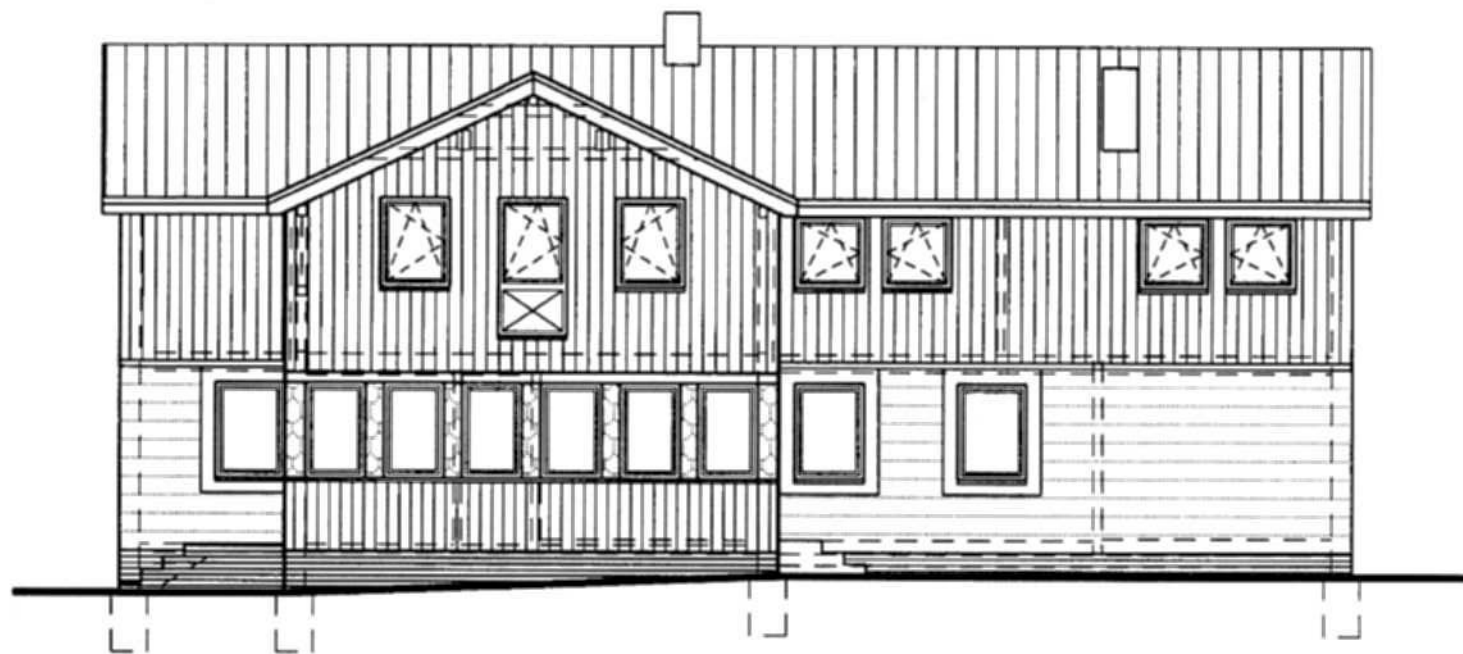
SÜD-WEST-ANSICHT
