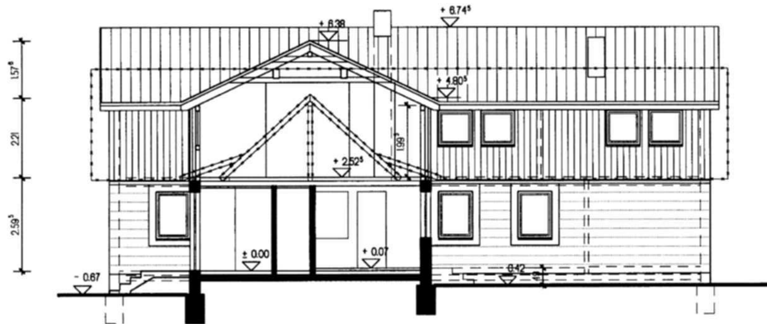
SCHNITT B-B
