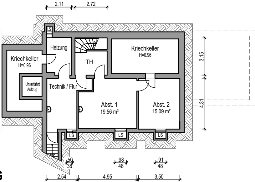
Grundriss WE4 UG
