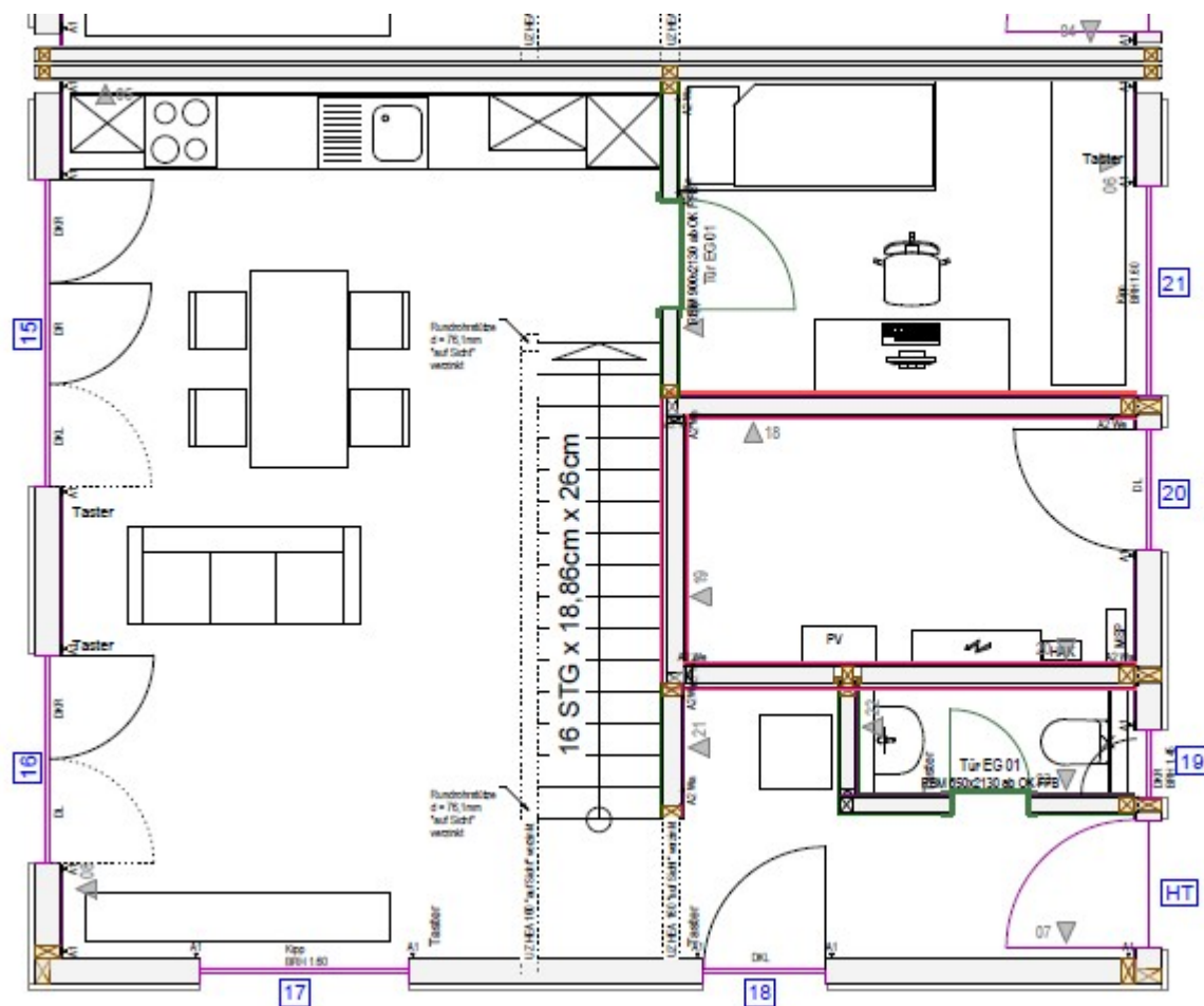
Erdgeschoss M: 1 : 50
