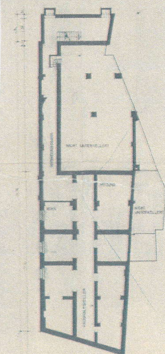
KELLERGEOSCHLOSS BESTAND
