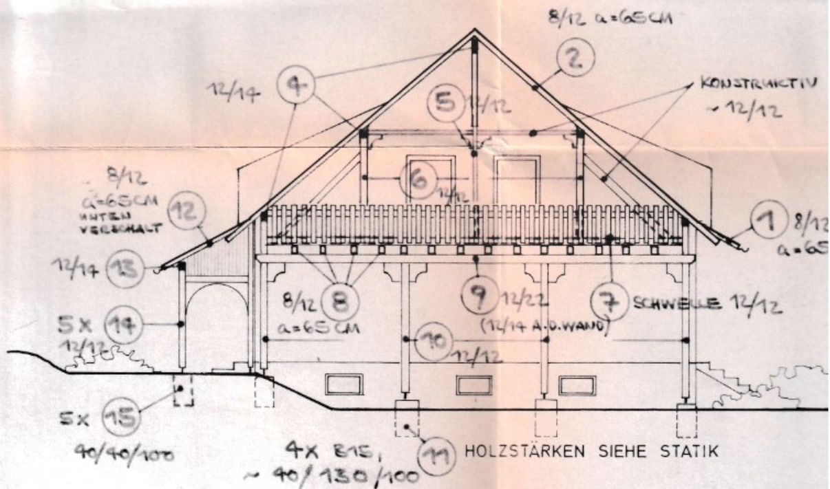
WESTANSICHT (neu)
