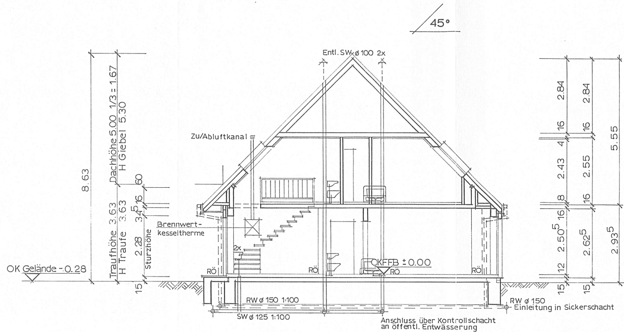
Querschnitt 1:100 EG Fussbodenhöhe 0.28 m über OK Gelände
