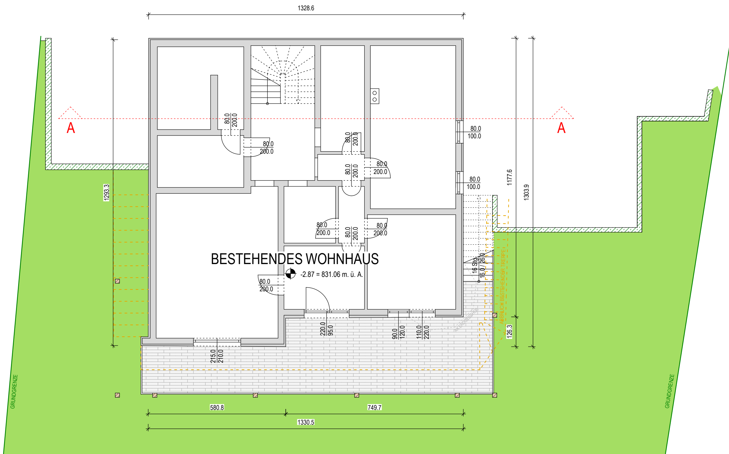
GRUNDRISS KELLERGEESCHOSS
