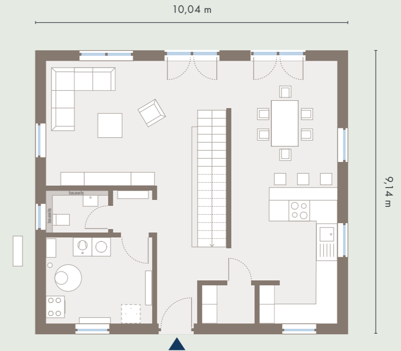
Erdgeschoss 75,82 m 2
