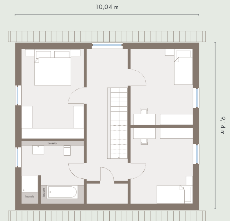
Dachgeschoss 74,48 m 2
