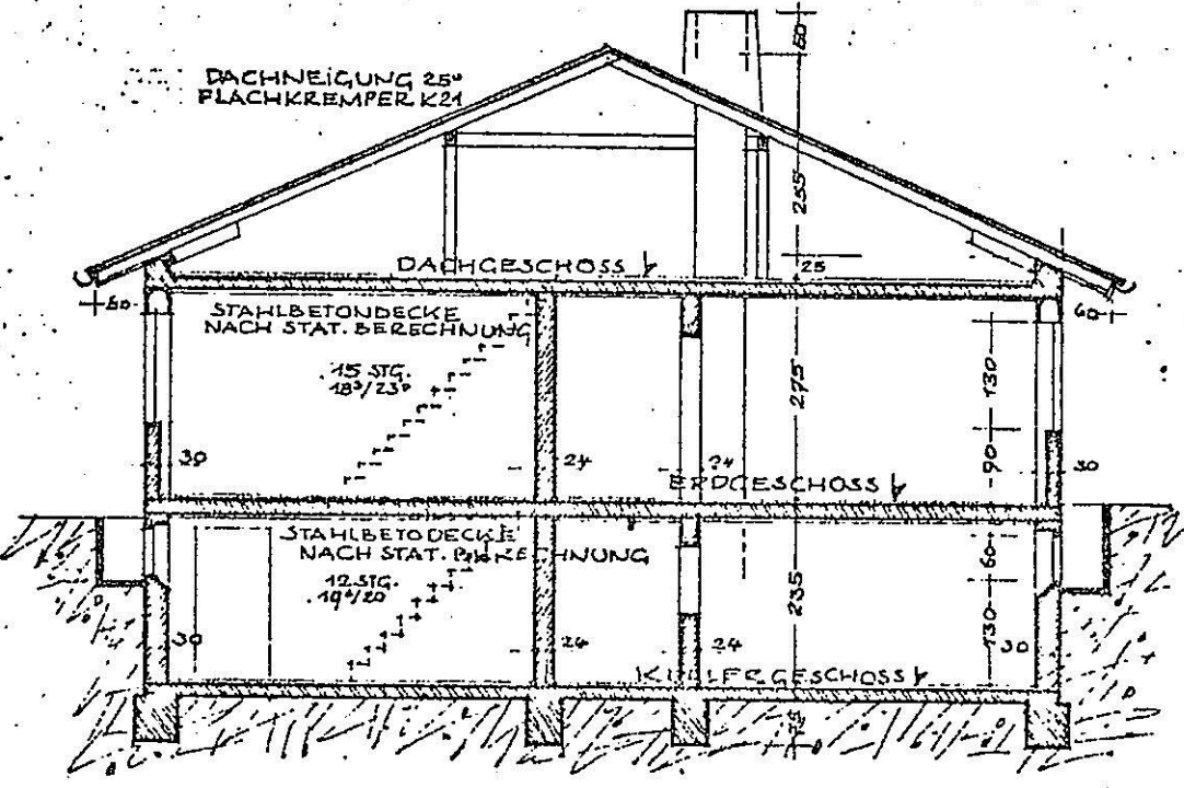
QUERSCHNITT A-B
