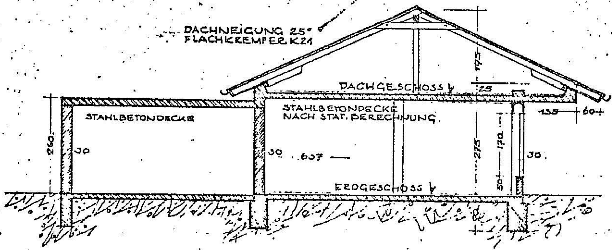
QUERSCHNITT C-D
