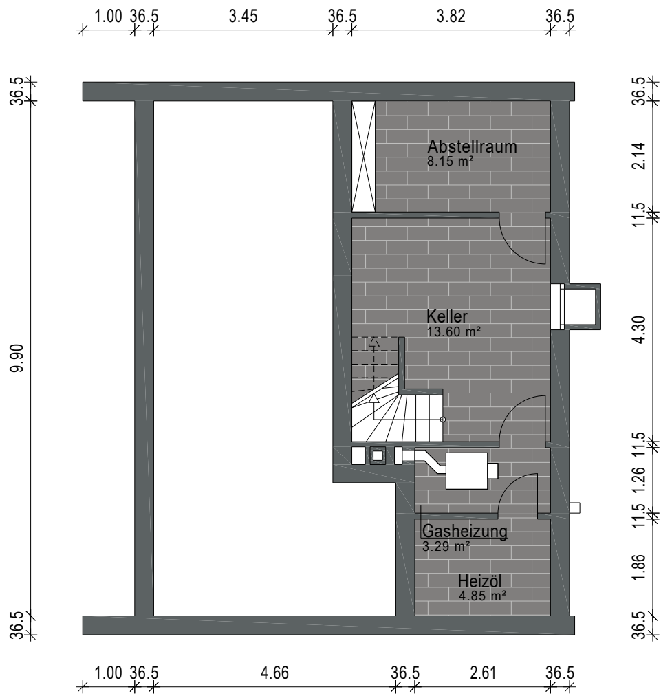
Kellergeschoss
