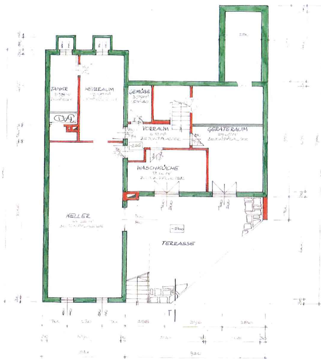
KELLERGESCHOSS
