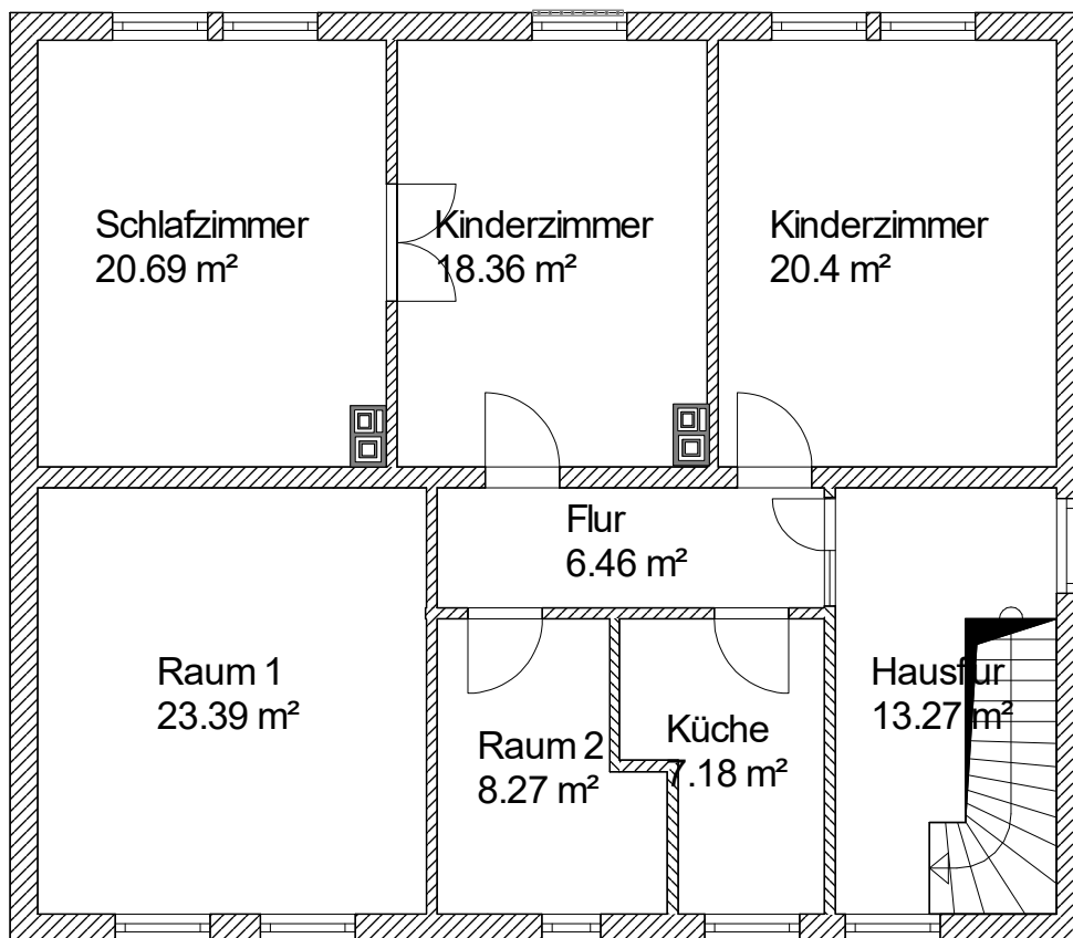
2.Obergeschoss
