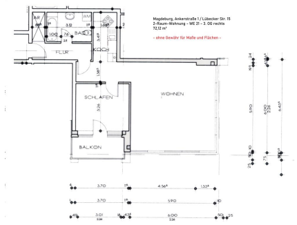
Grundriss
