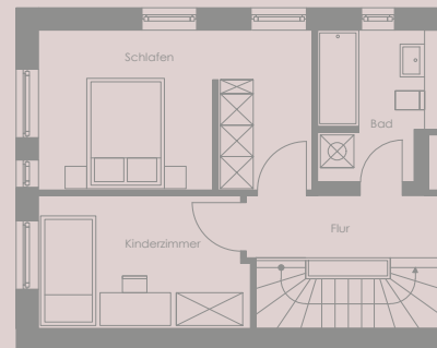
2. OBERGESCHOSS
