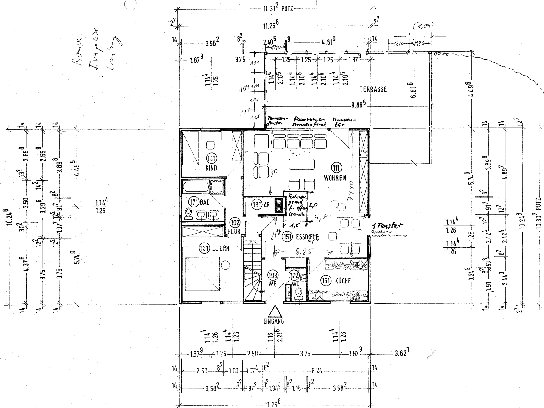
ERDGESCHOSS
