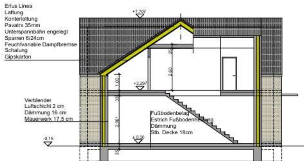
Schnitt B-B
