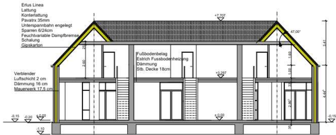
Schnitt A-A
