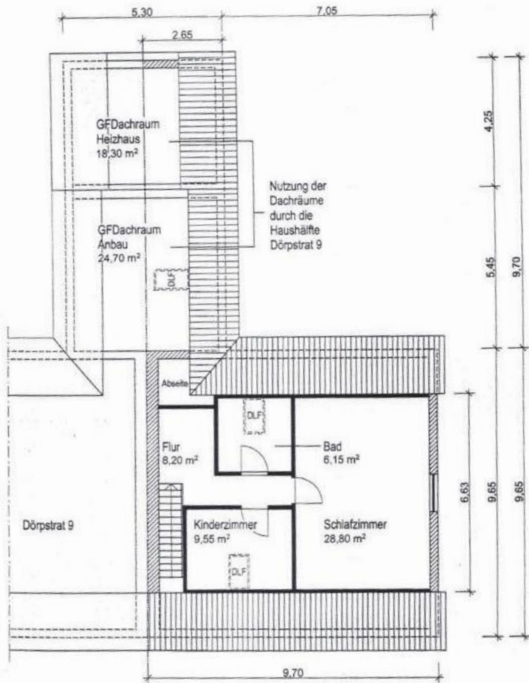
Grundriss DG Doppelhaushälfte o.M.
