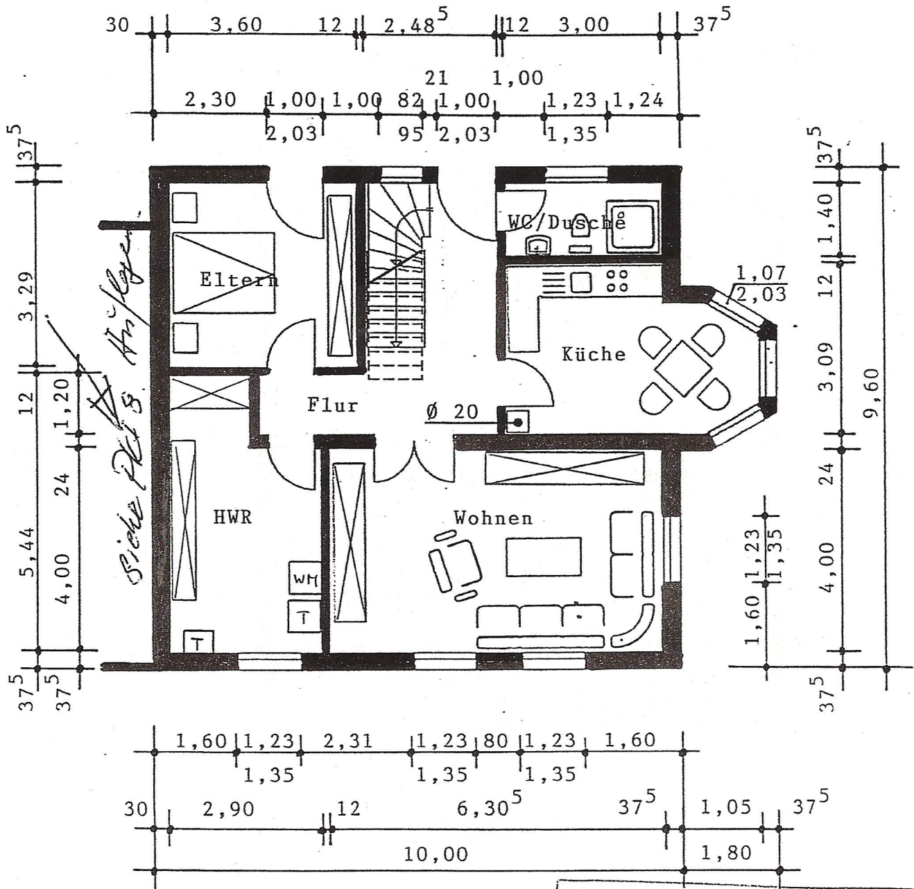
Erdgeschoßgrundriß M. 1:100
