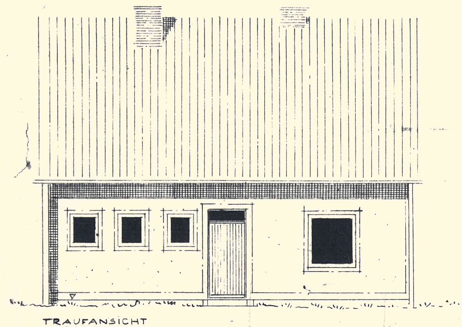
TRAUFANSICHT
