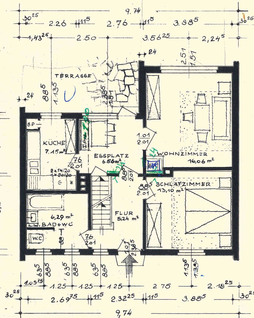
ERDGESCHOSS
