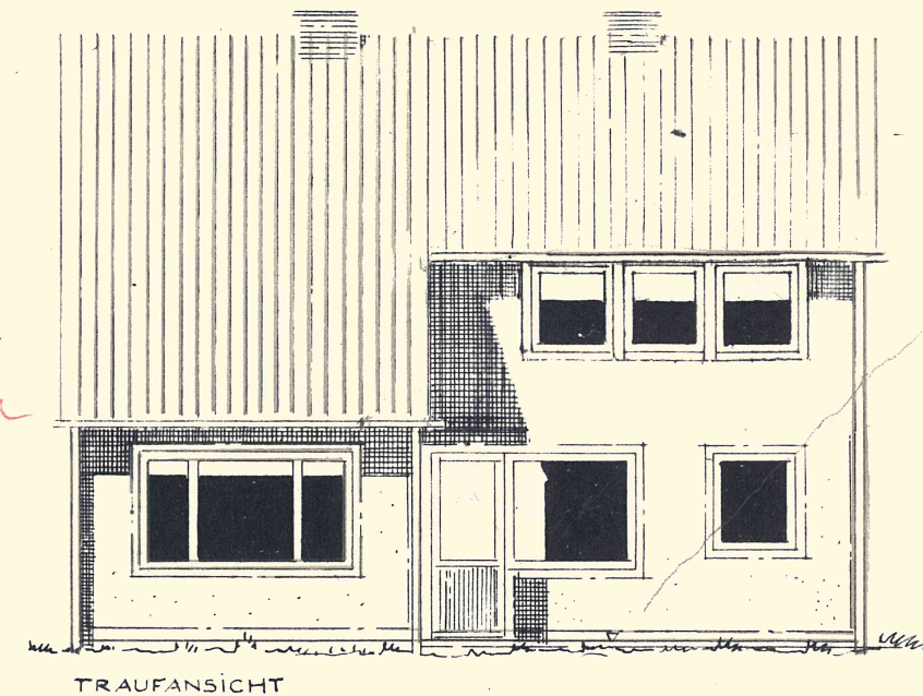
TRAUFANSICHT
