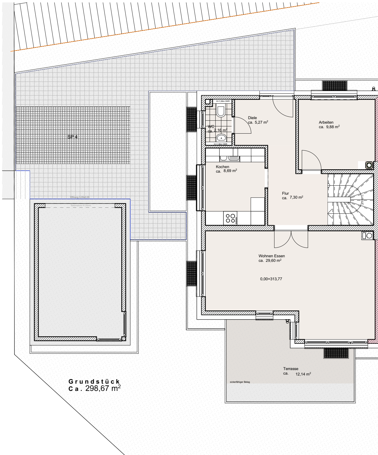
Grundriss EG M1:100
