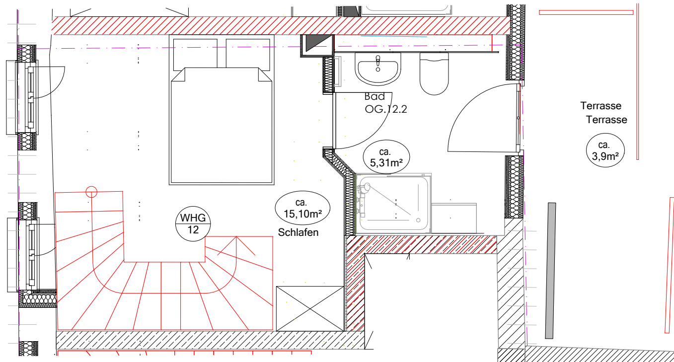
Dachgeschoß
