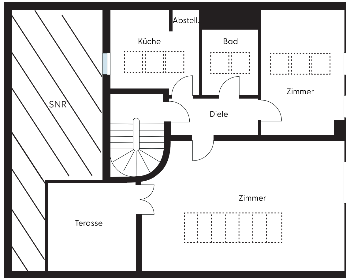
Ist Grundriss
